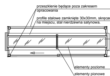
18 KONSTRUKCJA WSPORCZA POD PÓŁKI W GABLOCIE 1:50
