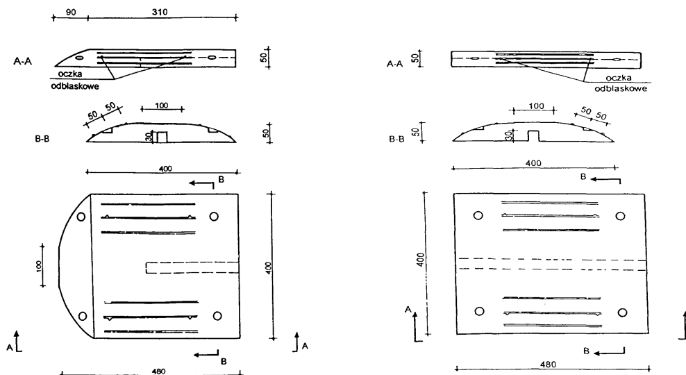
Rys. 3. Prógi typu listwowego długości 900 mm i wysokości 50 mm
