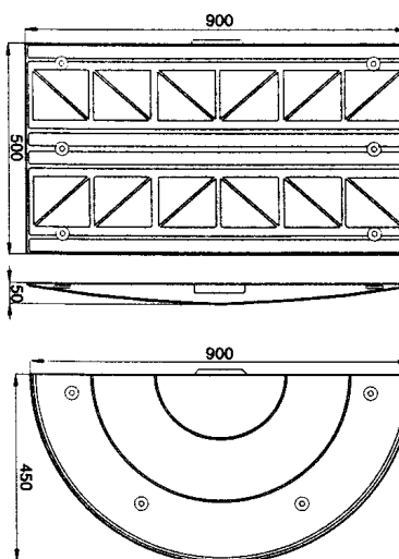
Rys. 3. Prógi typu listwowego długości 900 mm i wysokości 50 mm
