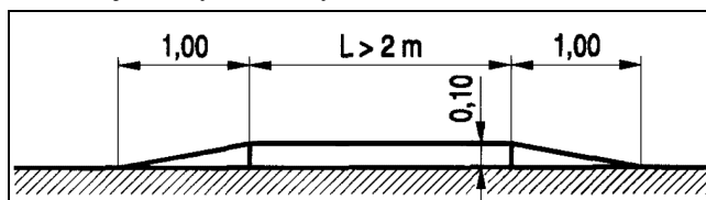
Rys. 4. Przekrój podłużny liniowego progów zwalniającego listwowego o ograniczonej prędkości przejazdu 18 \div 20 km/h (U-16d)
