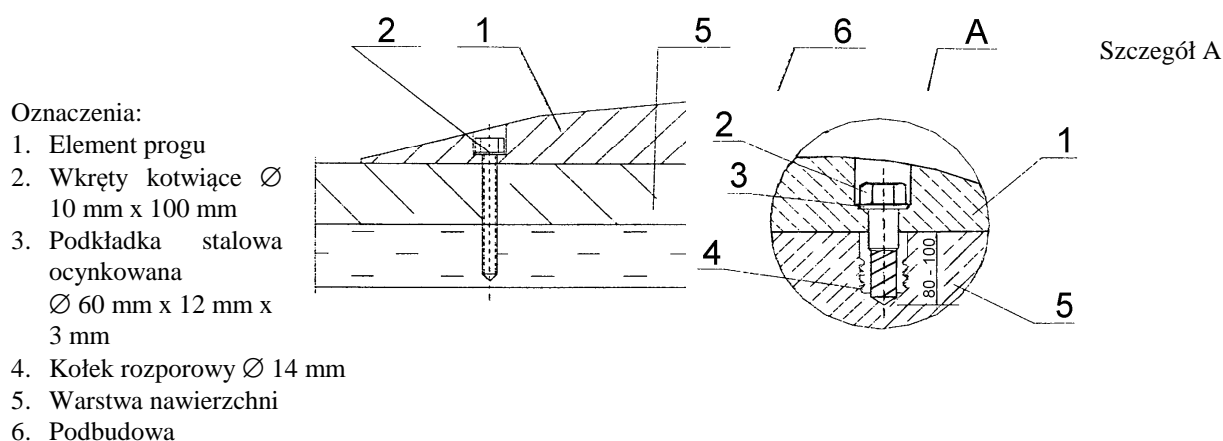
Rys. 4. Przykład umocowienia progu do nawierzchni jezdni
