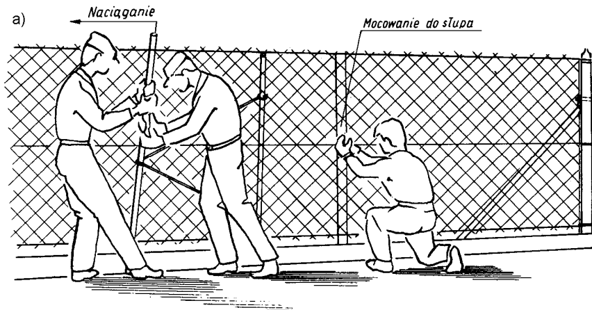
Rys. 9. Przykłady mocowania siatki do linii usztywniających (wg [6])
