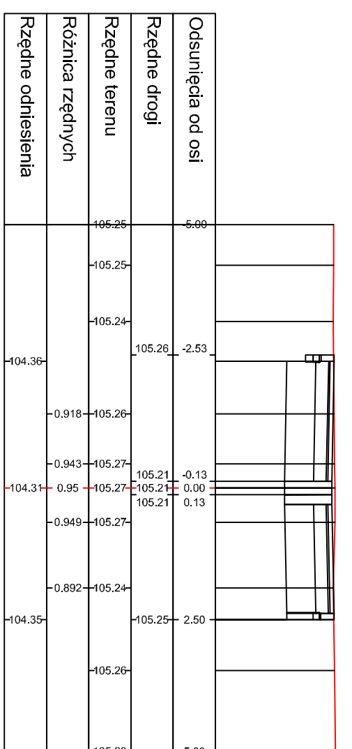
Ul. Łagodna PK 0+220.000
