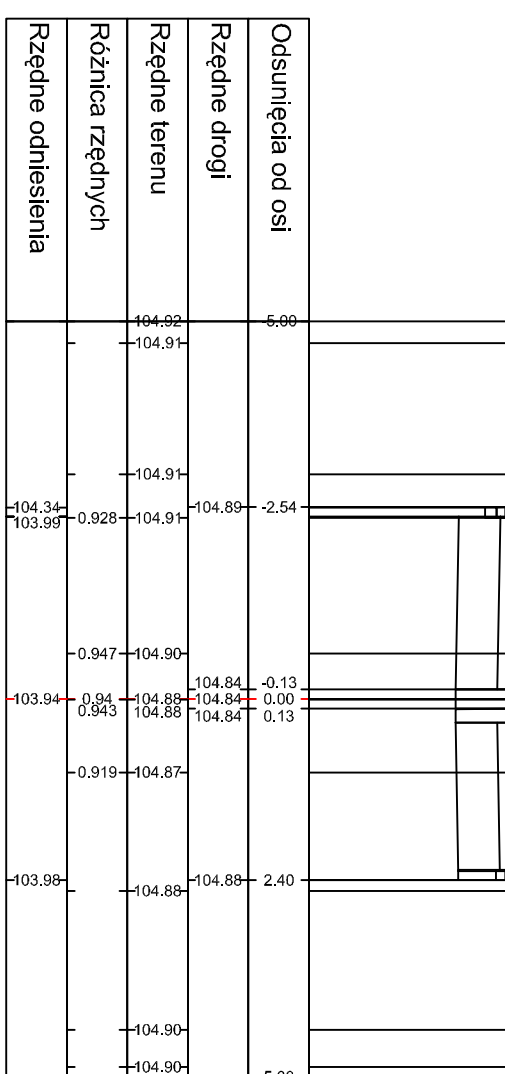
Ul. Łagodna PK 0+160.000
