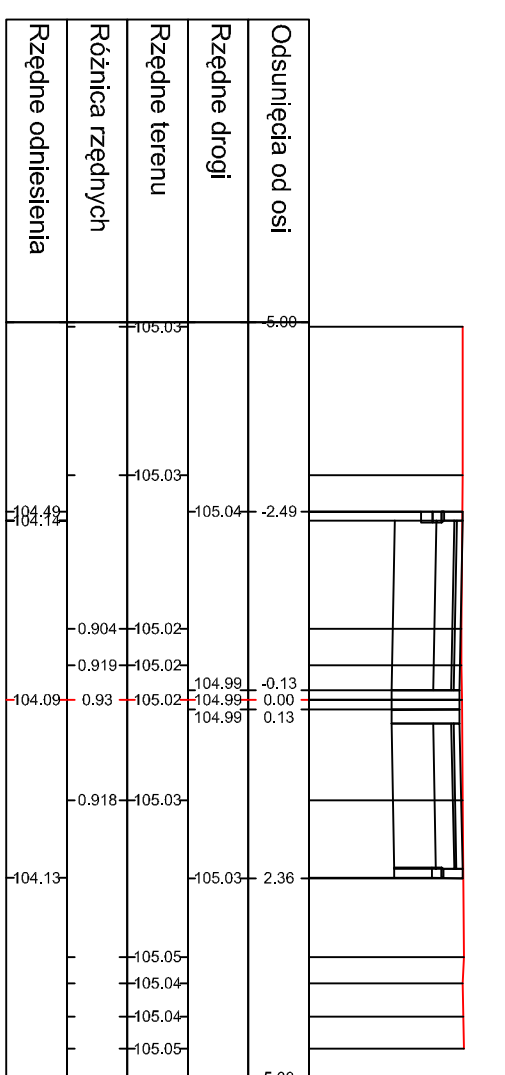
Ul. Łagodna PK 0+140.000
