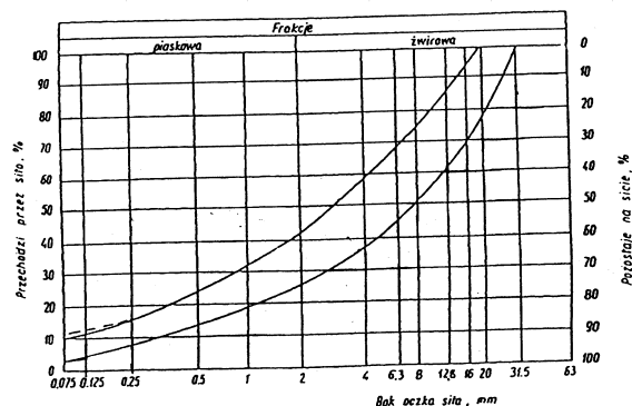
Rys. 1. Pole dobrego uziarnienia kruszyw dla podbudowy
