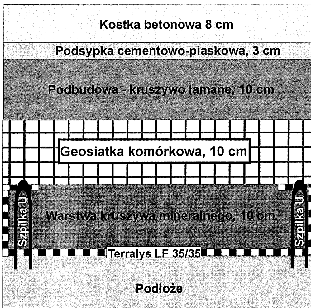
Rys.15. Uproszczony schemat układu warstw konstrukcji i podłoża wzmocnionego geosiatką komórkową
